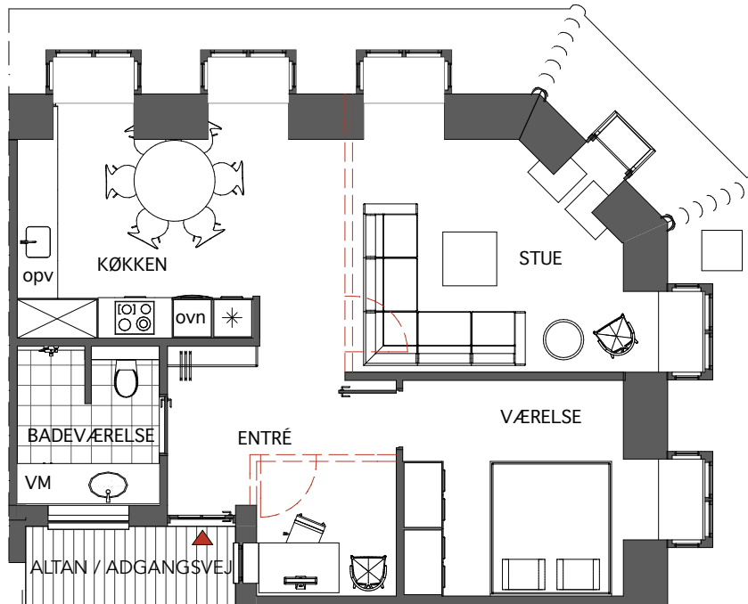
PLAN, MÅL 1:100
